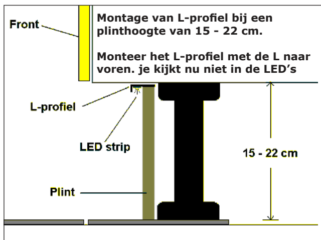
afb.1 montage plintverlichting bij hoge plint
