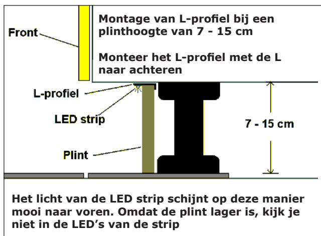
afb.4 montage plintverlichting bij lage plint
